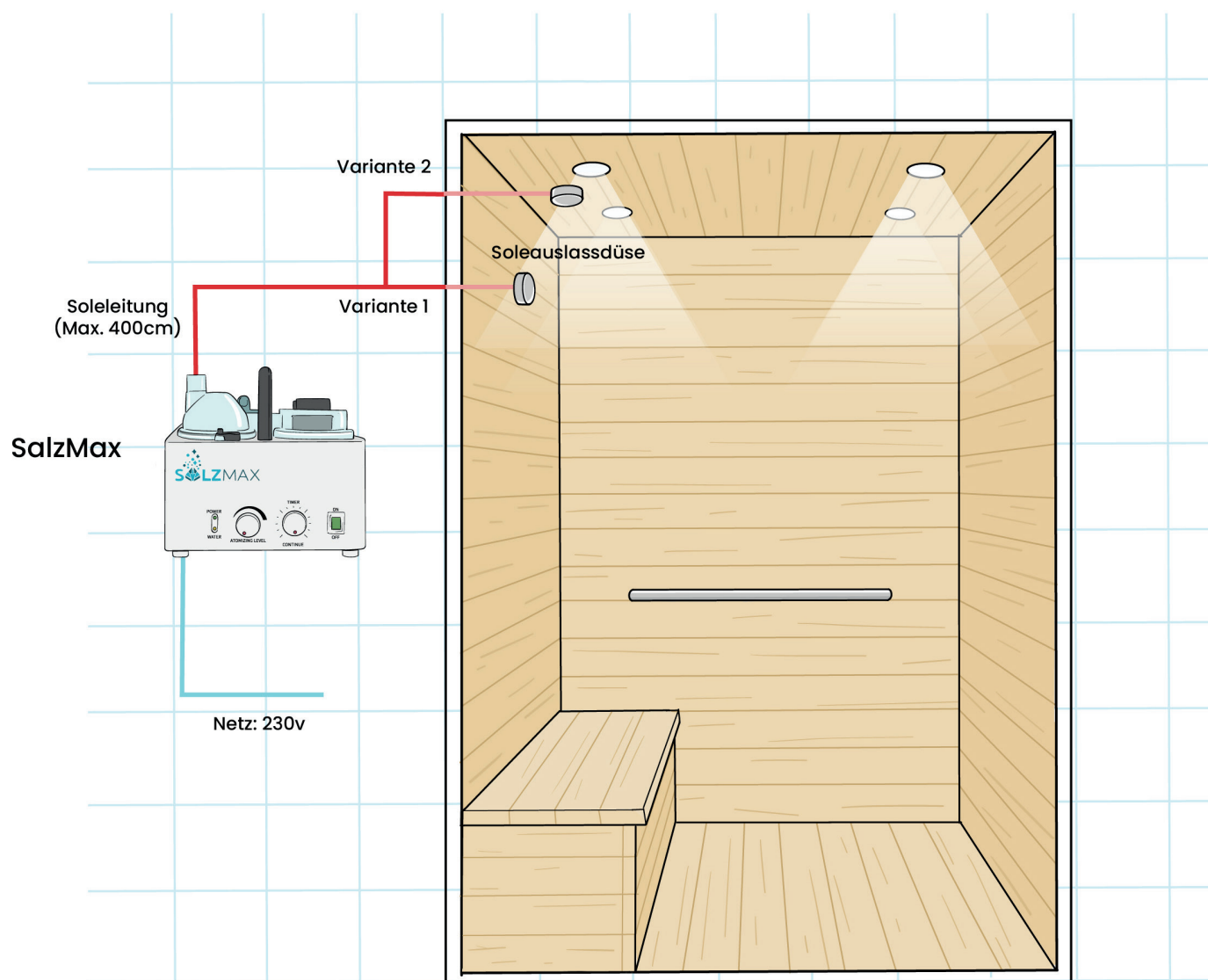
Abbildung 3: Einbau Sauna/Infrarotkabine
