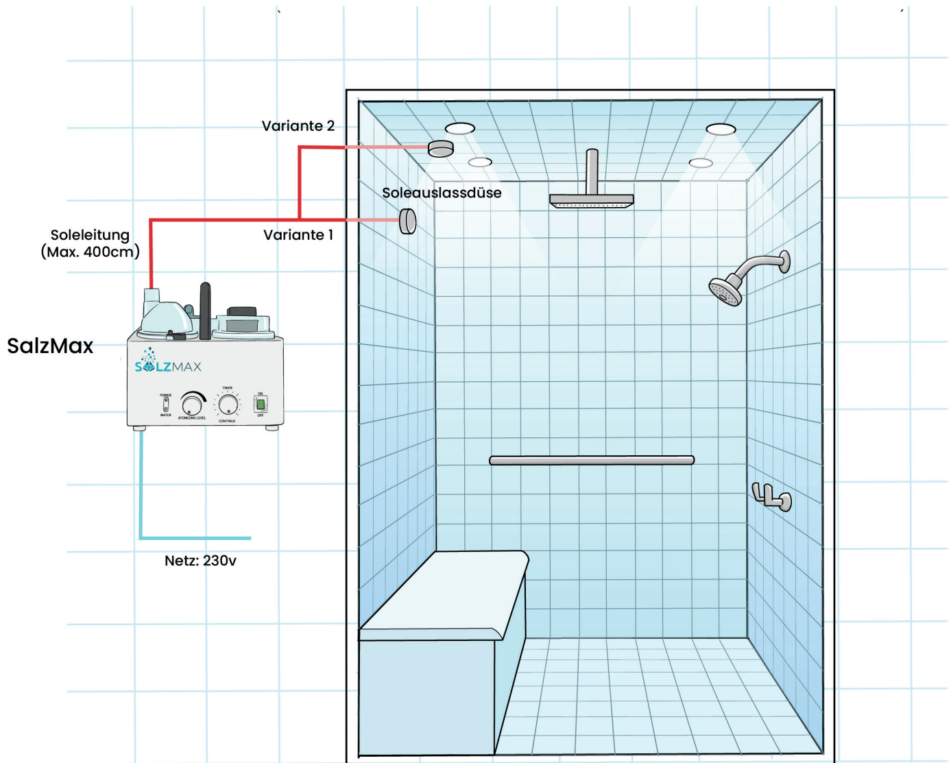
Abbildung 2: Einbau Dampfbad/Dampfdusche
