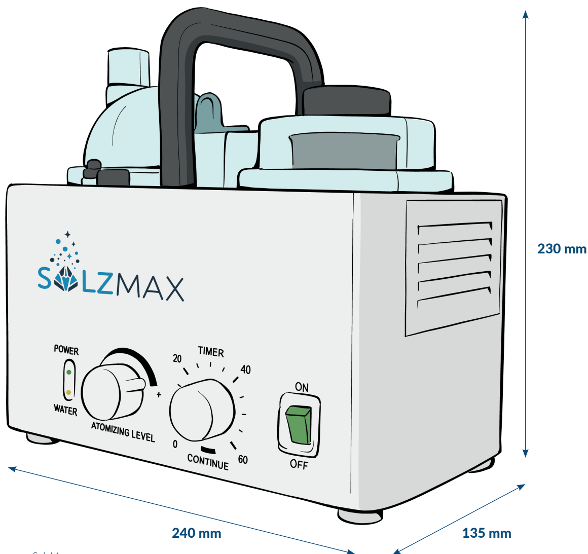
Abbildung 1: Abmessungen SalzMax
