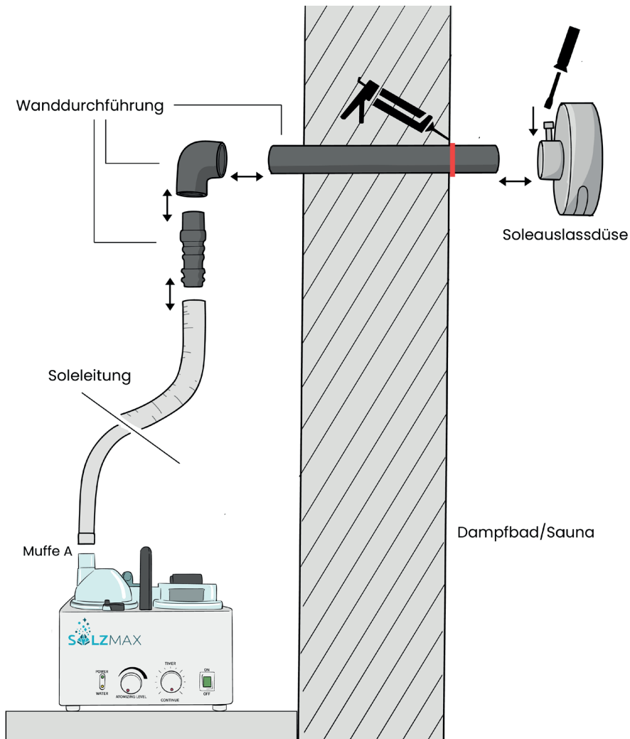
Abbildung 4: Wanddurchführung Soleauslassdüse
