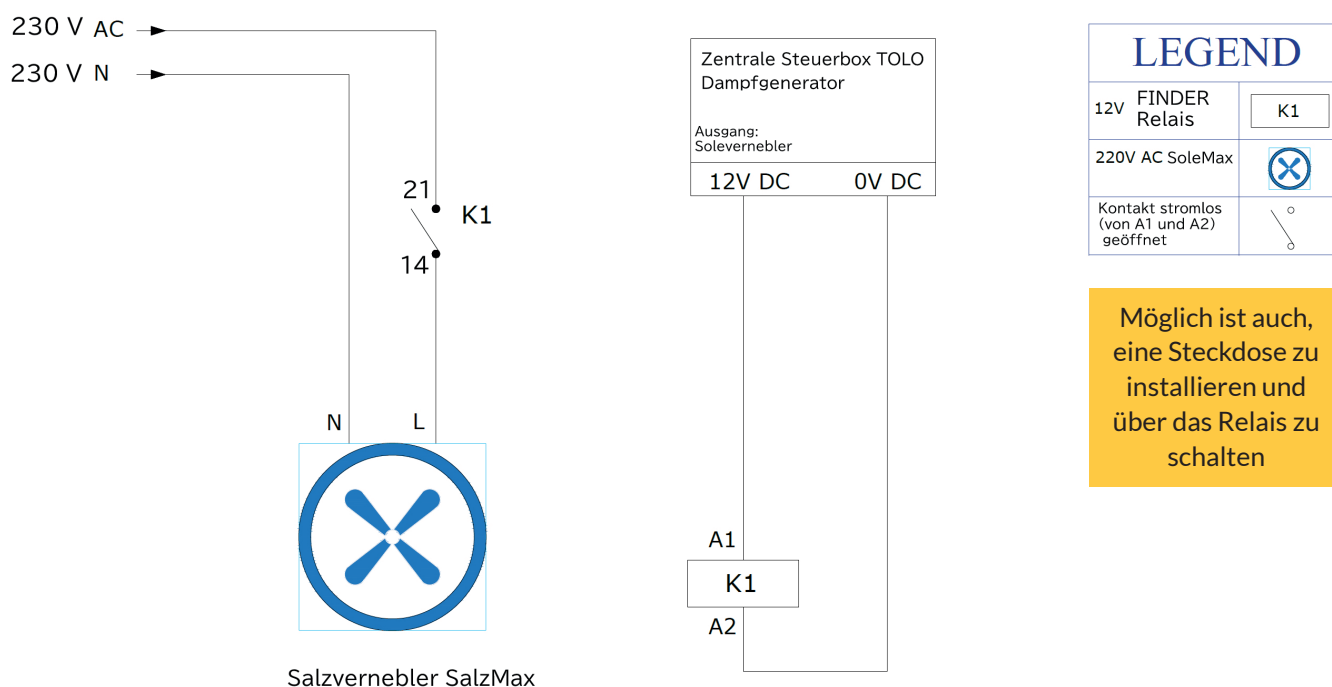
Abbildung 5: Verbinden von SalzMax und TOLO Dampfgenerator
